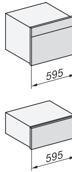
Einbau DG, DGM, DGC XL, ESW7x20, Skizze,
